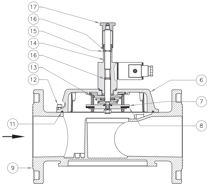
fig. 1 DN 65 - DN 80
