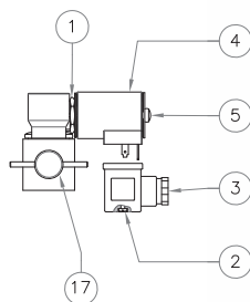
Bobina vista dall'alto Top view of the coil Bobina vista desde arriba
