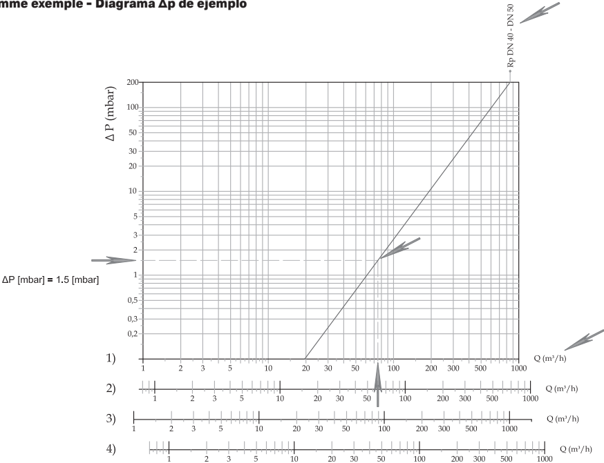
Diagramma perdite di carico FM-FGM filtraggio 50 \mu m (calcolato con P_1 = 0 mbar) FM-FGM pressure drop diagram filtering 50 \mu m (calculated with P_1 = 0 mbar) Diagramme de perte de charge FM-FGM filtrage 50 \mu m (calculé avec P_1 = 0 mbar) Diagrama de pérdidas de carga filtración 50 \mu m (calculado con P_1 = 0 mbar)
