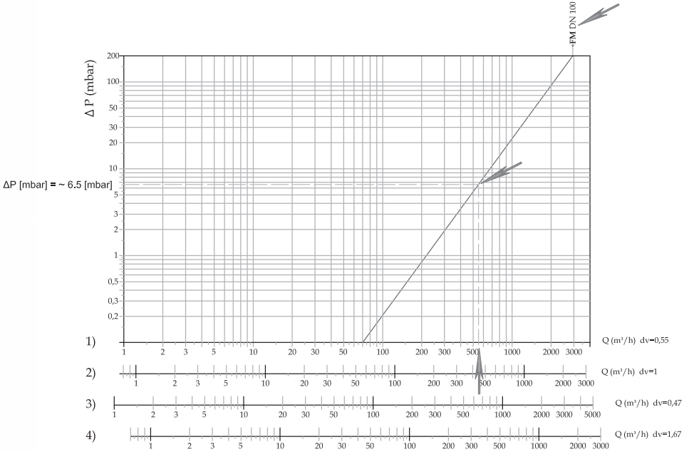
Diagramma perdite di carico FM filtraggio 50 µm (calcolato con P_1 = 0 mbar) FM pressure drop diagram filtering 50 µm (calculated with P_1 = 0 mbar) Diagramme de perte de charge FM filtrage 50 µm (calculé avec P_1 = 0 mbar) Diagrama de pérdidas de carga filtración 50 µm (calculado con P_1 = 0 mbar)
