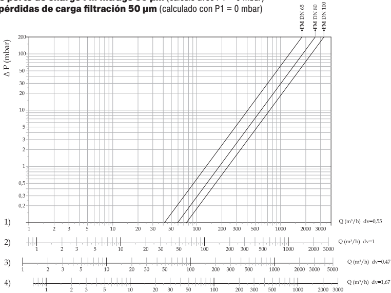
Diagramma perdite di carico FM filtraggio 50 µm (calcolato con P_1 = 0 mbar) FM pressure drop diagram filtering 50 µm (calculated with P_1 = 0 mbar) Diagramme de perte de charge FM filtrage 50 µm (calculé avec P_1 = 0 mbar) Diagrama de pérdidas de carga filtración 50 µm (calculado con P_1 = 0 mbar)
