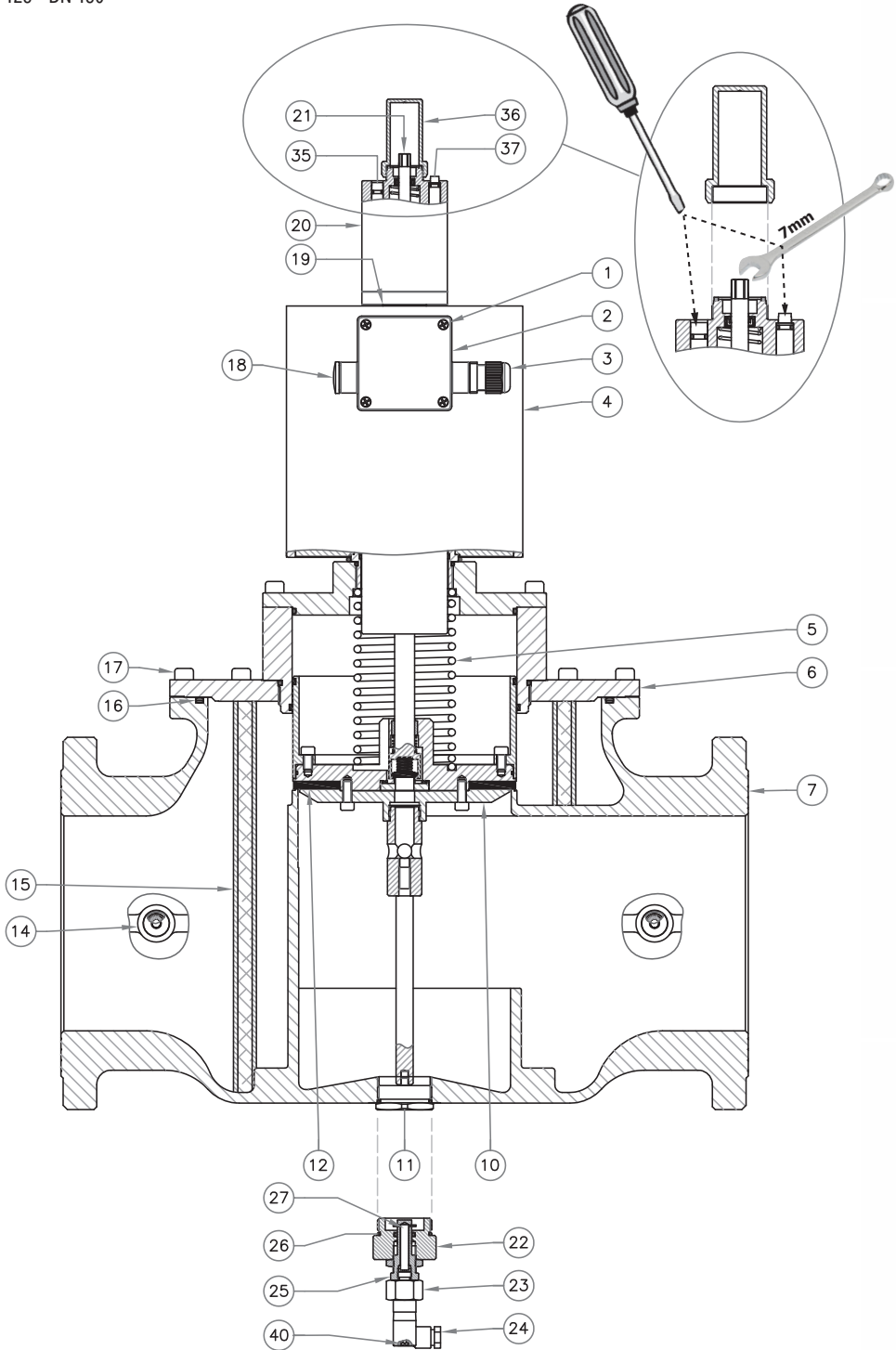
fig. 4 DN 125 - DN 150
