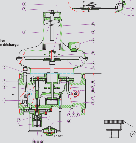
fig. 1 senza sfioro without relief valve sans vanne de décharge sin alivio
