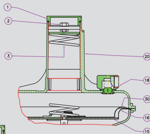
FIG N° 1-2 (STANDARD DN 65 ÷ 100)
